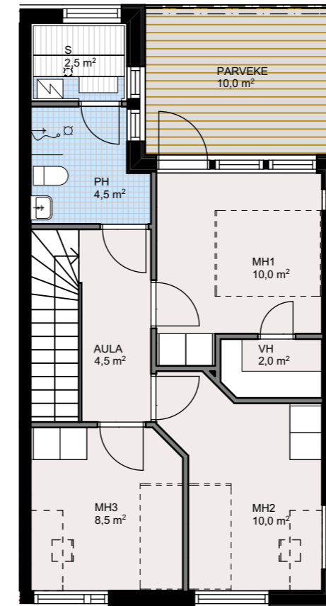
2.krs
