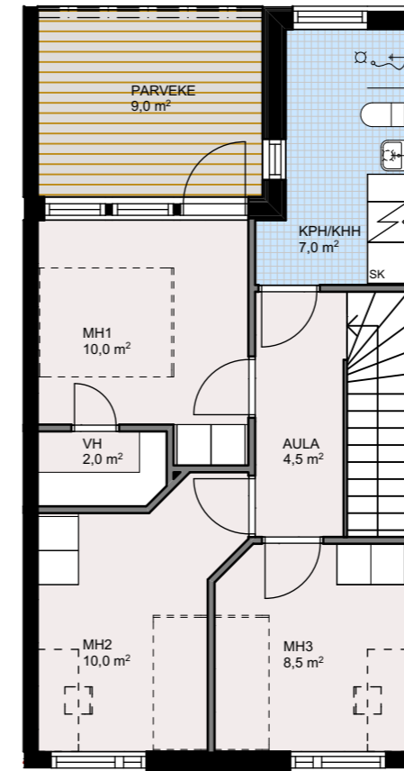
2.krs
