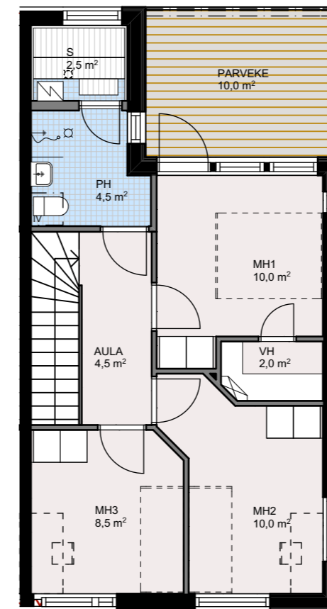
2.krs
