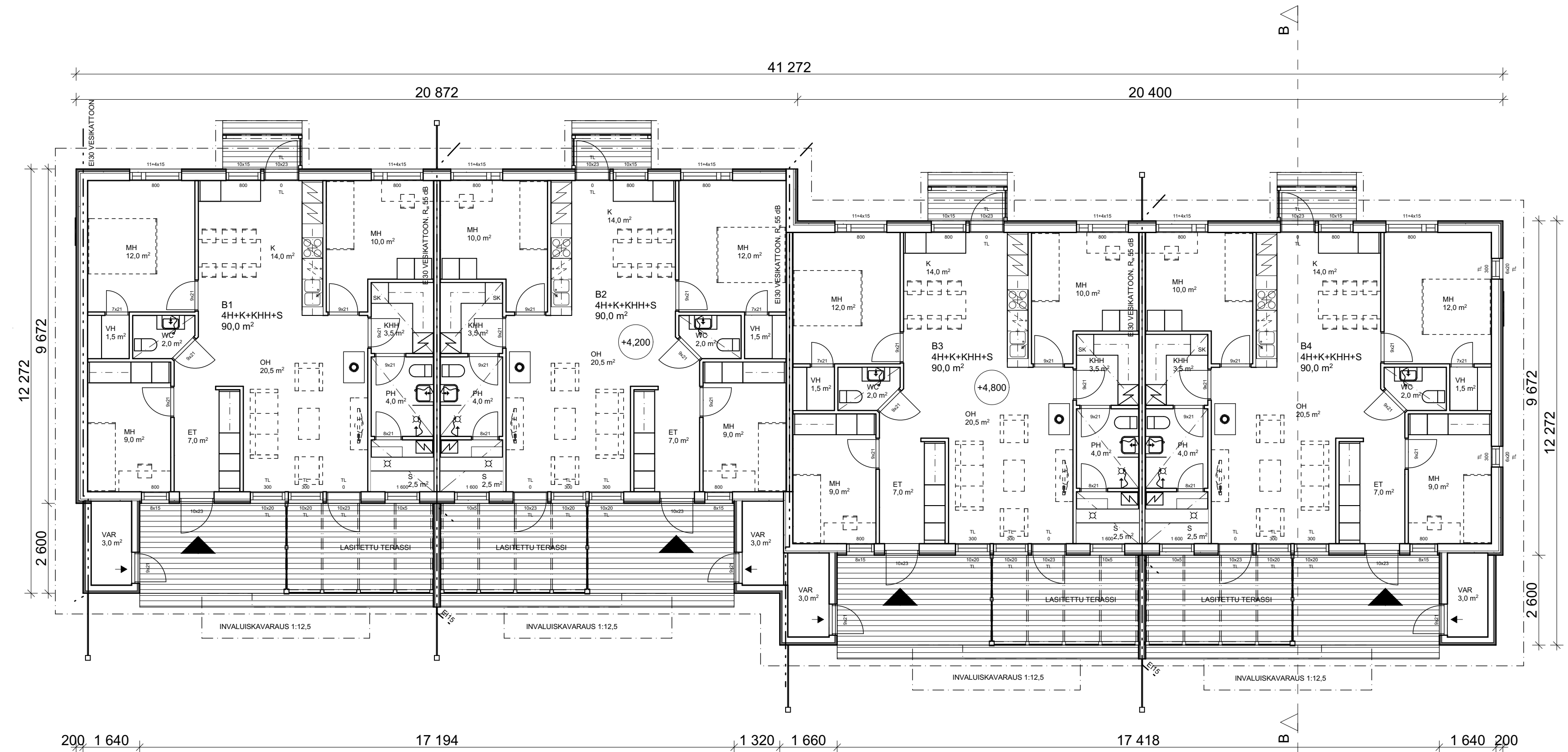
POHJAPIIRUSTUS RAK2
